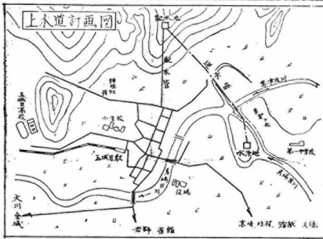
上水道計画 〇給水区域 旧五城目町、旧大川村全域 〇給水人口 10,500人 〇最大給水量 1,890立方メートル(10,400人) 〇総事業費 5,500万円 〇工事期間 昭和34~36年度の三年継続 今年融資をまつて着工、34、35、36年の起債を 見合水年度内通水を目標に計画を進めている。
