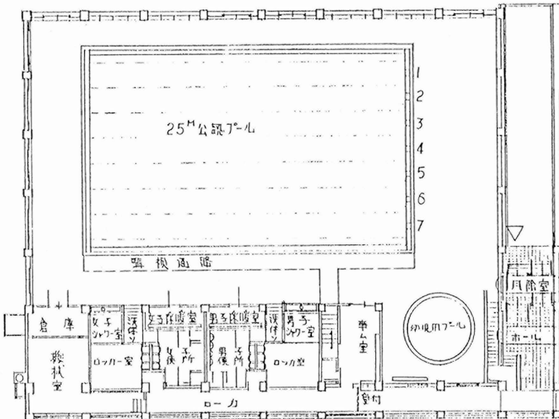
屋内温水プール 1階平面図 (縮尺:1/300)
