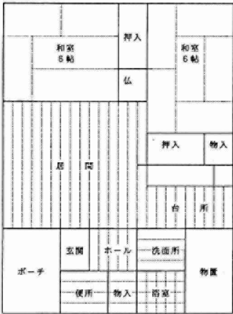
第2種住宅Bタイプ — 2戸— (61.27㎡)
