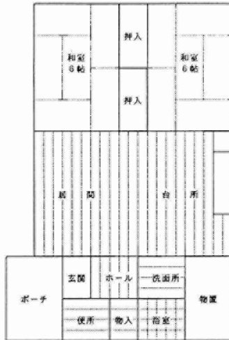
第2種住宅Aタイプ — 2戸— (61.27㎡)
