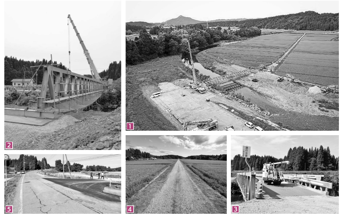
1 県道秋田八郎湯線と門前町内を結ぶ仮橋の供用を開始。 2 大型クレーンを使用して仮橋を設置。 3 9月17日の供用開始後、門前町内の住民や付近の耕作の方々が仮橋を利用。 4 迂回路となる農道は、今後拡幅舗装工事を実施します。 5 馬場目浄水場の向かい付近が迂回路と県道との合流部。
